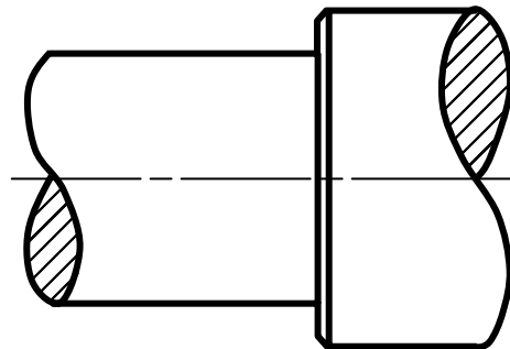
شافت
