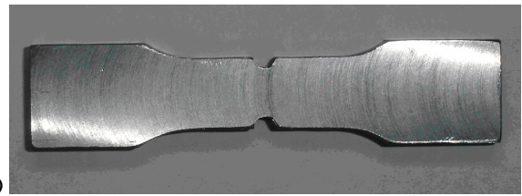
شکل ۲- نمونه شیاردار تهیه شده برای تعیین پارامترهای آسیب
