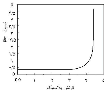
شکل ۱۱- نمودار رشد تنش سه محوره در المان
